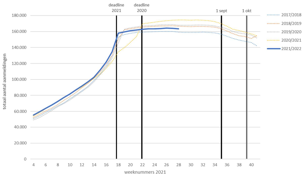
Figuur 1: Cumulatief aantal aanmeldingen voor hbo opleidingen (associate degree, bachelor of master) per week voor de laatste vijf jaar inclusief aanmelddeadlines, start studiejaar (1 sept) en verwerkingsdeadline inschrijvingen (1 okt).
